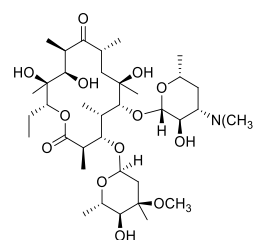
Erythromycin A
