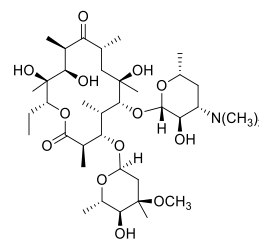
Erythromycin A
