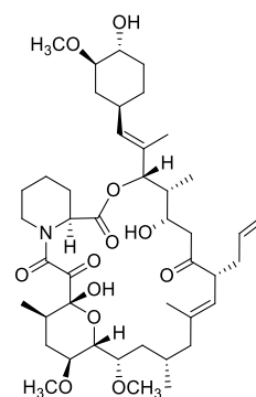
Tacrolimus
