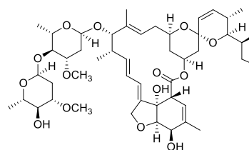
Avermectin B1a
