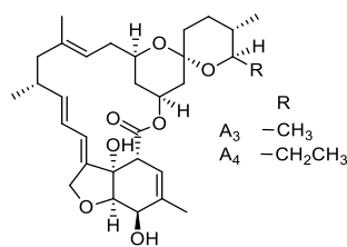
Milbemectin
