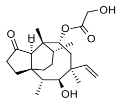
Pleuromutilin
